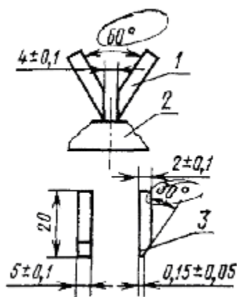
1 - электрод; 2 - испытуемый образец; 3 - конец электрода скруглен
