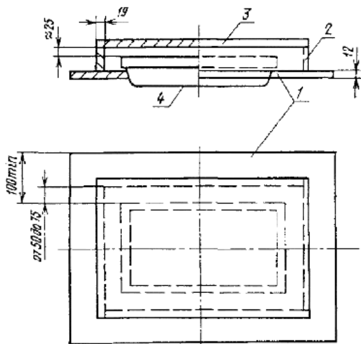
1 - основа, 2 - боковая стенка, 3 - верхняя стенка, 4 - испытуемый светильник
