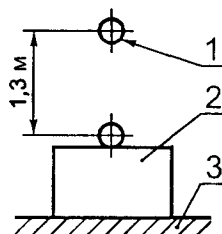
1 - стальной шарик; 2 - светильник; 3 - опорная поверхность
