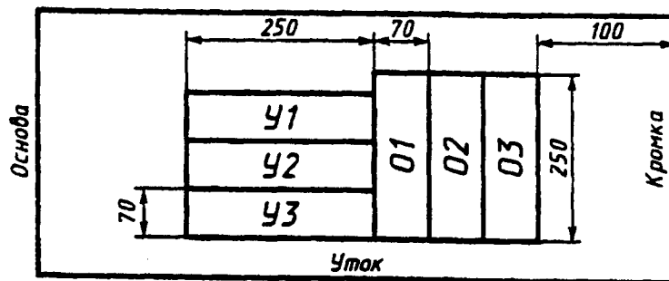
Y 1 , Y 2 , Y 3 — заготовки уточных пробных полосок; O 1 , O 2 , O 3 — заготовки основных пробных полосок
